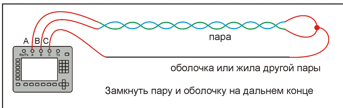
Схема подключения
