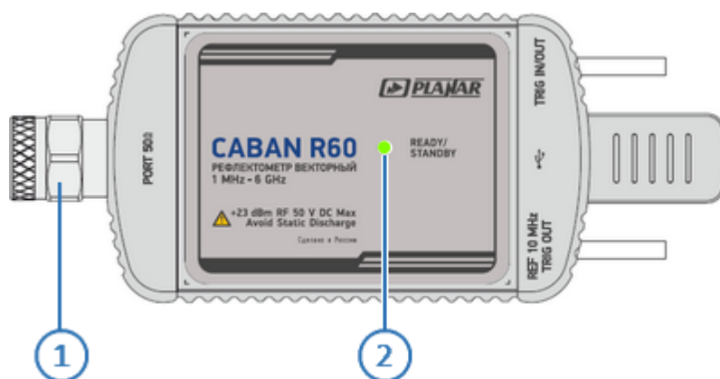
Рисунок 12 – Обратная сторона CABAN R60
