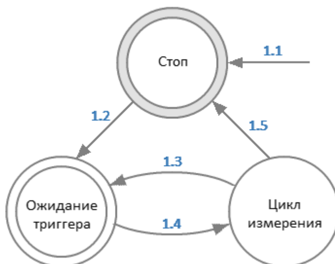
Рисунок 53 — Состояния и переходы измерителя
