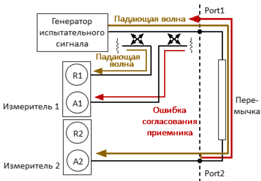
Рисунок 87 – Ошибка согласования приемника
