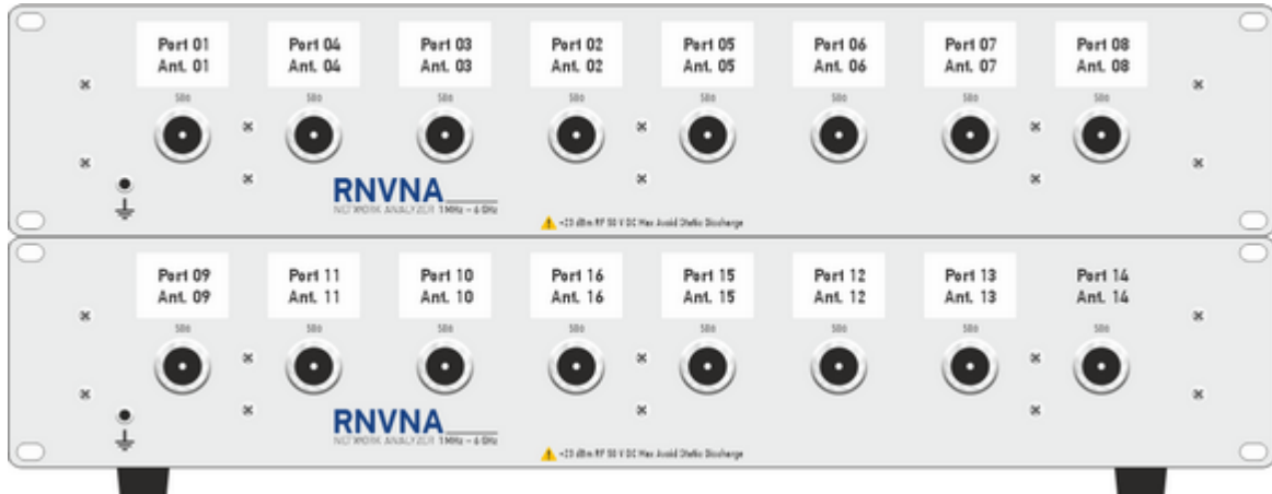
Рисунок 28 – Лицевая сторона измерителя RNVNA
