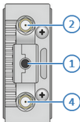
Рисунок 13 – Торцевая сторона CABAN R60
