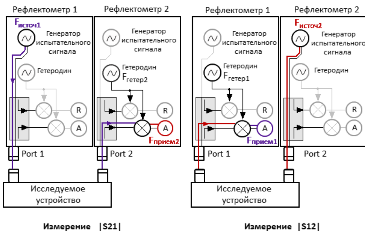
Рисунок 143 — Измерение S-параметров исследуемого устройства без подстройки частоты генераторов
