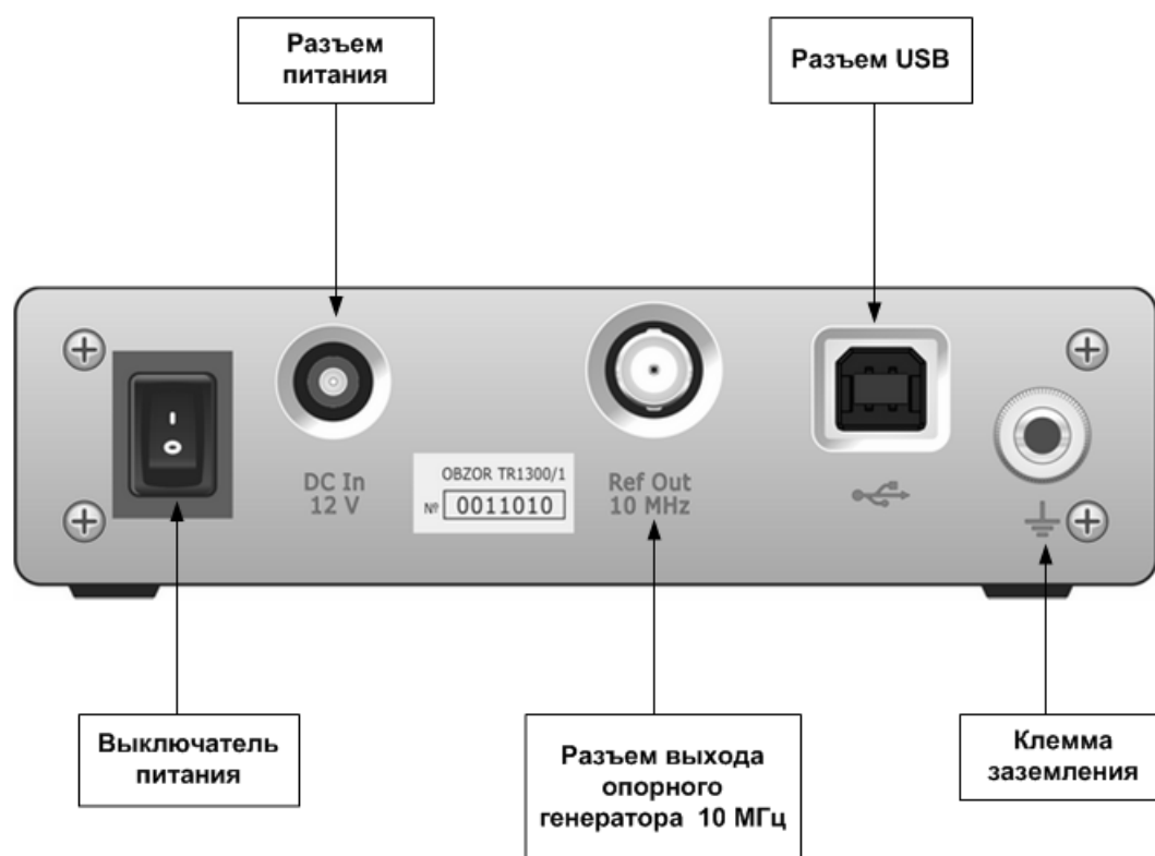
Рисунок 3.3. Задняя панель измерителя «Обзор TR1300/1»
