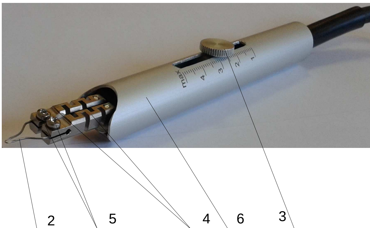
Рис.1.Инструмент с установленным V-образным электродом.
