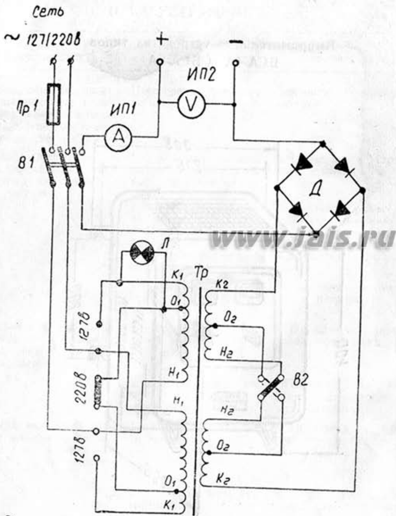
Схема переключения перемычек клет- мной панели трансформатора
