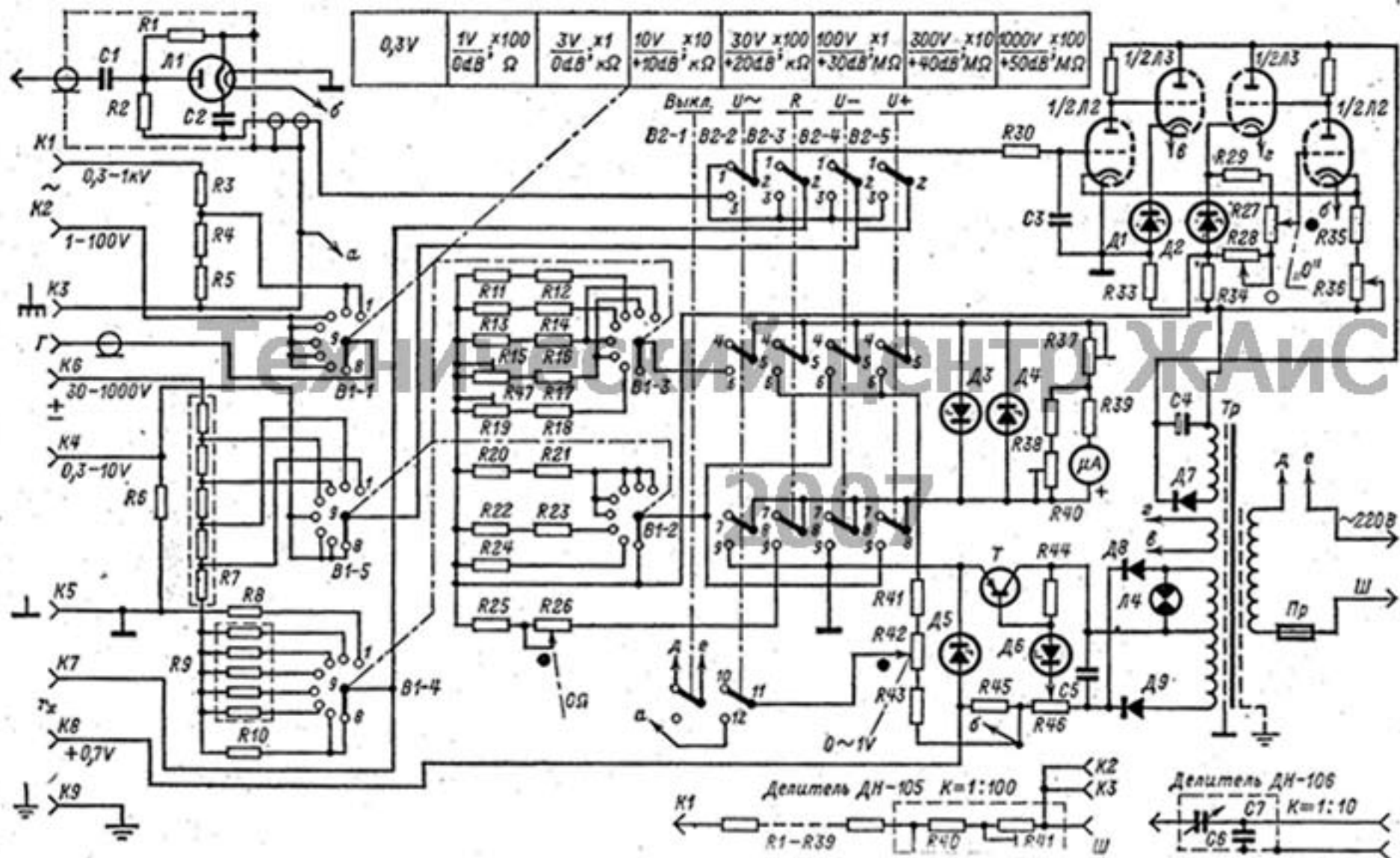
Электрическая принципиальная схема вольтметра ВК7-15.
