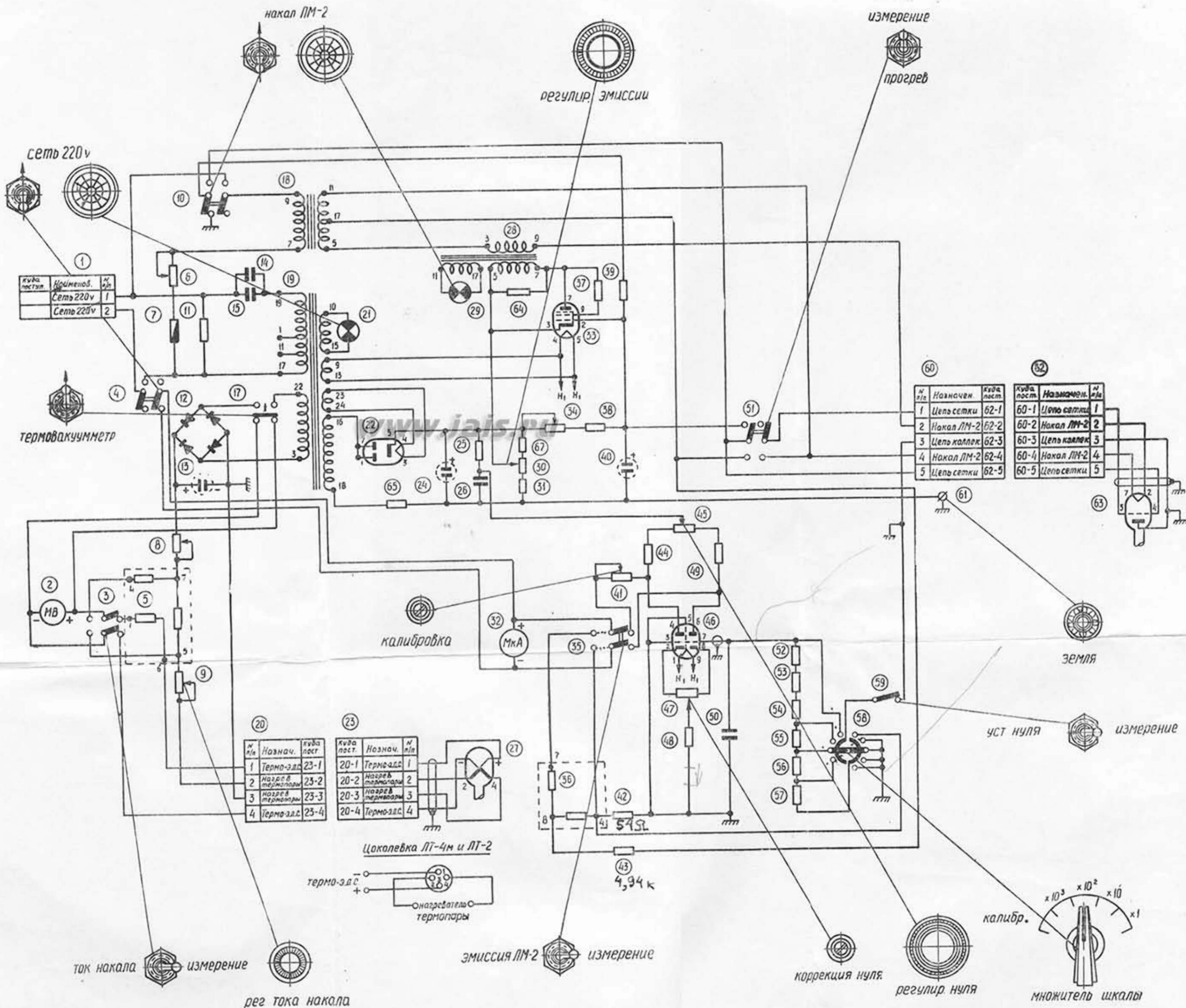
5. Принципиальная схема прибора ВИТ-1А.
