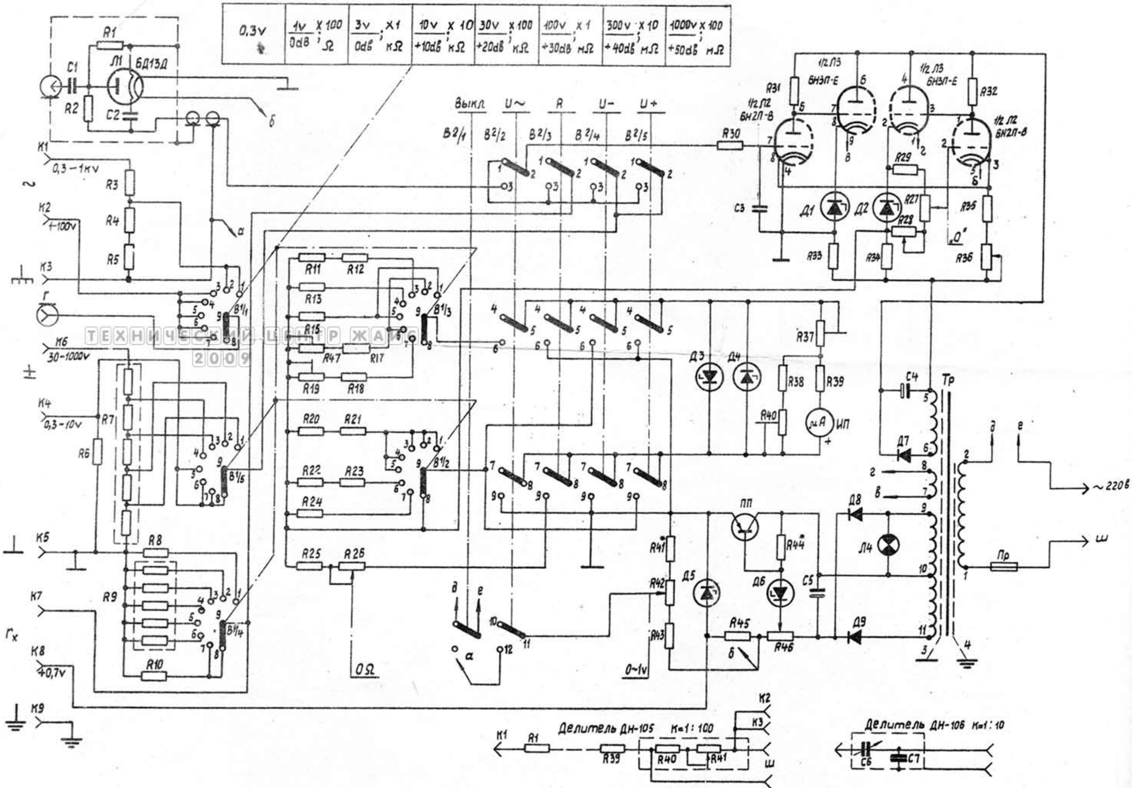
СХЕМА ПРИНЦИПИАЛЬНАЯ ЭЛЕКТРИЧЕСКАЯ
