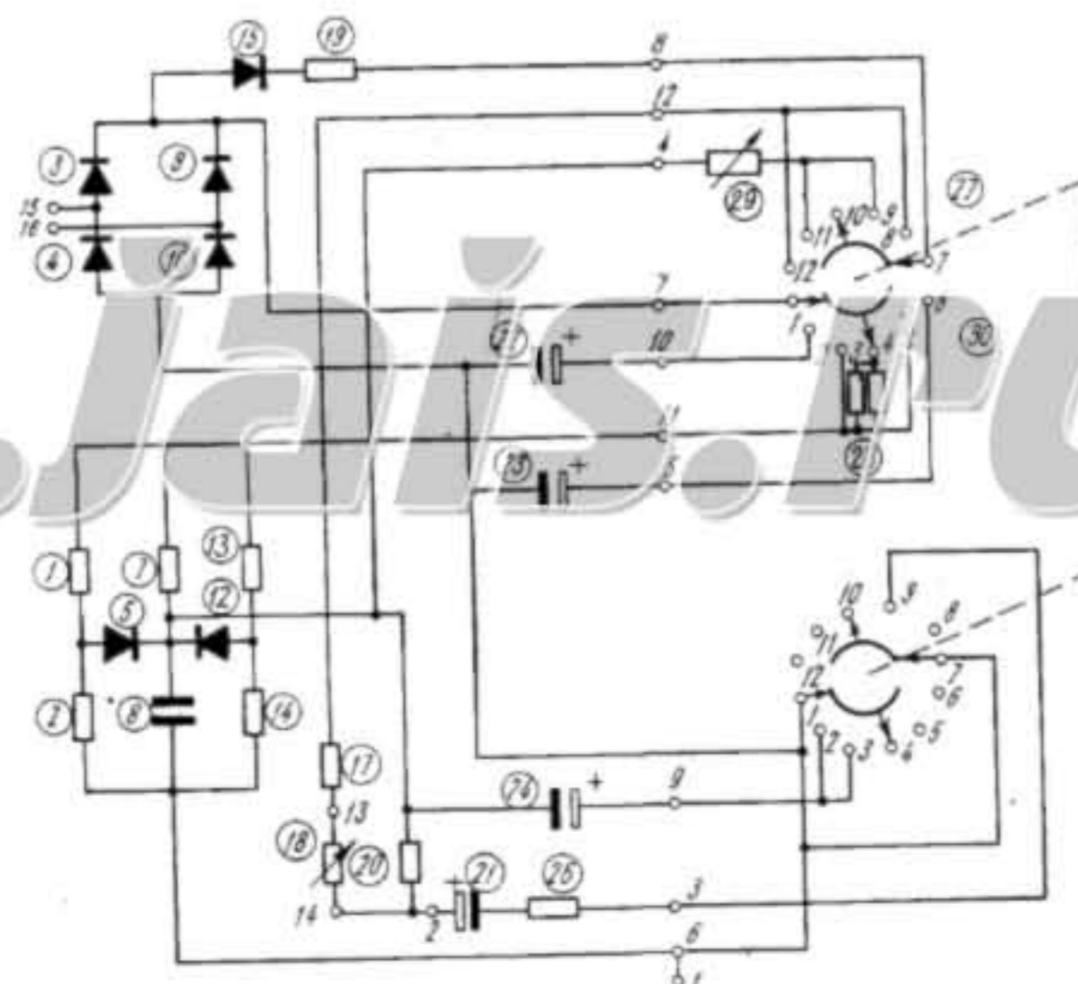
ПРИНЦИПАЛЬНАЯ ЭЛЕКТРИЧЕСКАЯ СХЕМА ВЫПРЯМИТЕЛЯ
