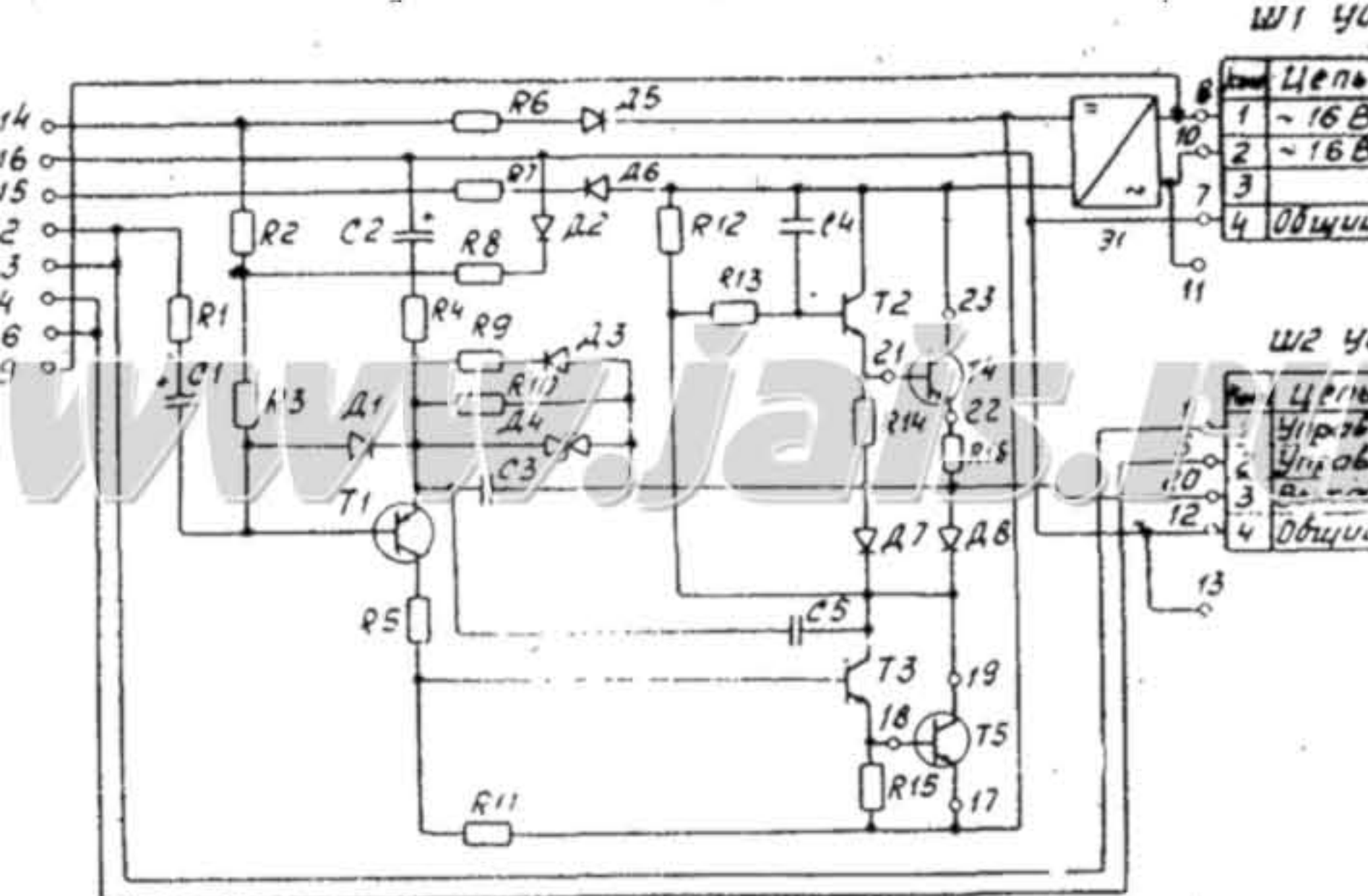
Усилитель оконечный
