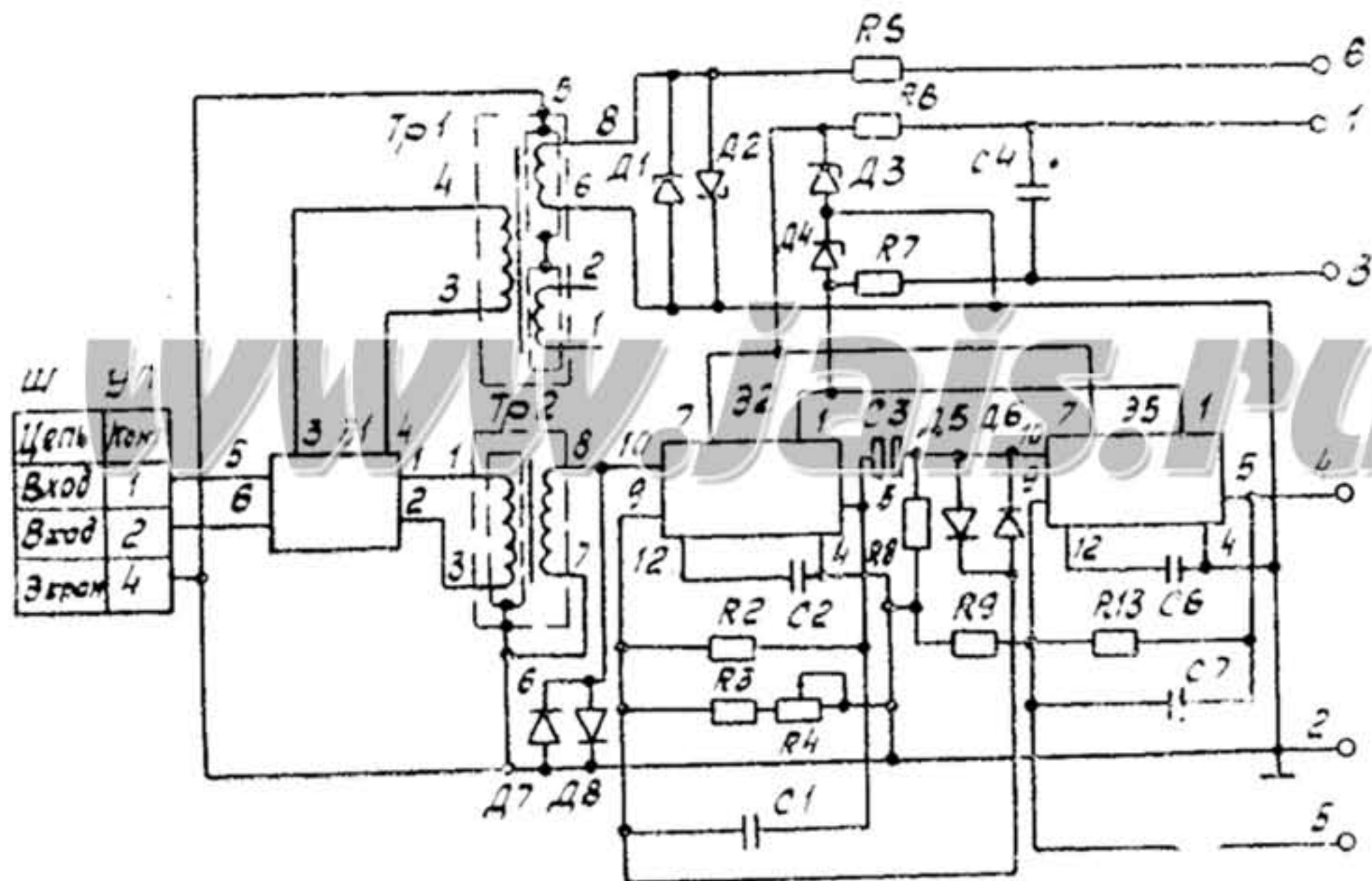
Усилитель предварительный
