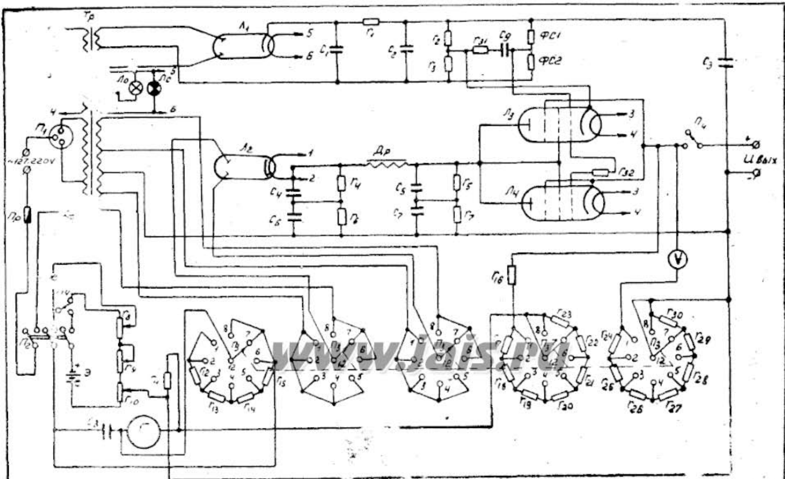
рис. 1. Принципиальная схема стабилизированного выпрямителя УИЗВ
