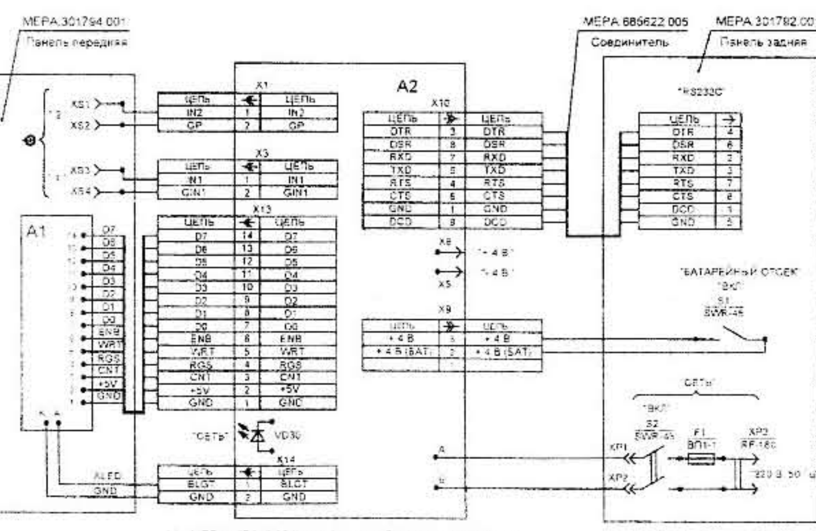
Схема электрическая принципиальная прибора
