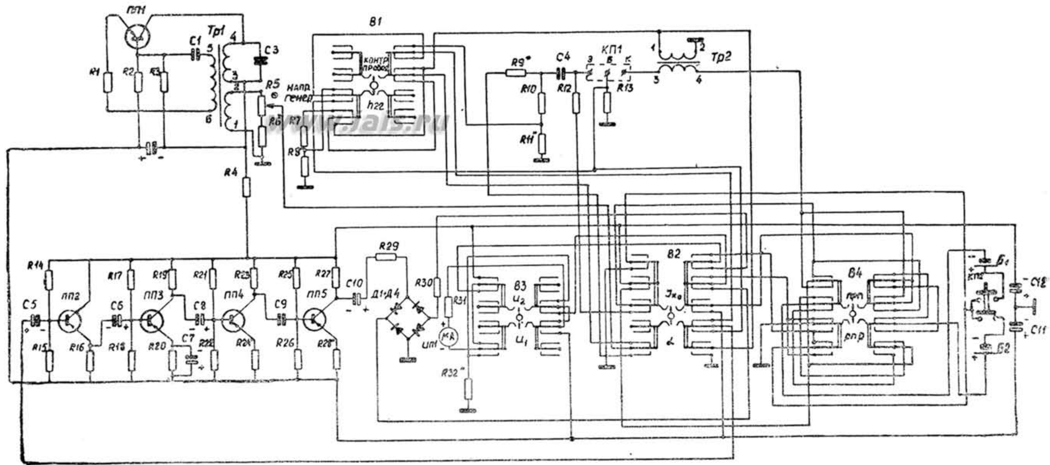
Рис. 6. Принципиальная схема.
