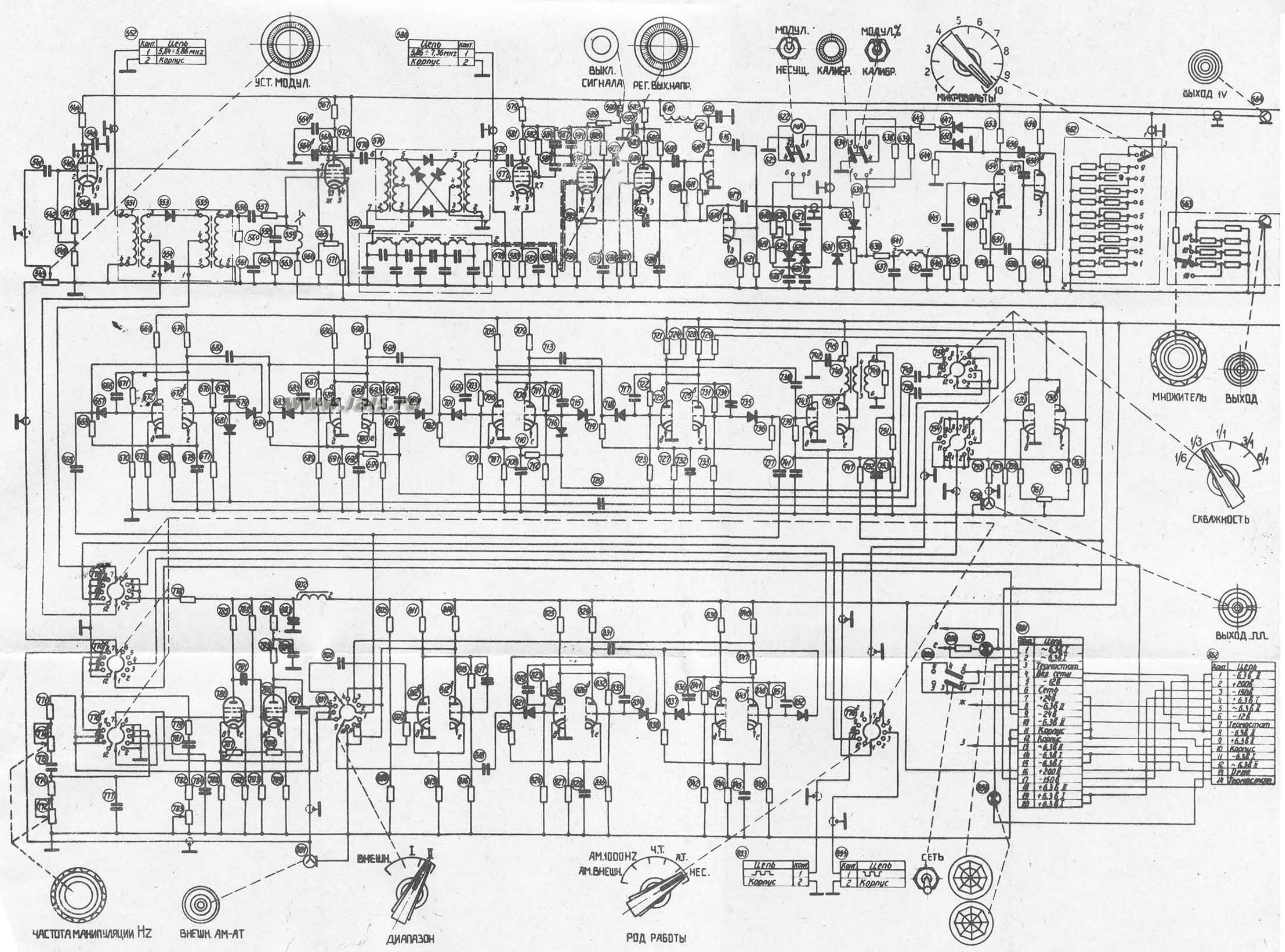
15. Принципиальная электрическая схема блока манипулятора Г4-46
