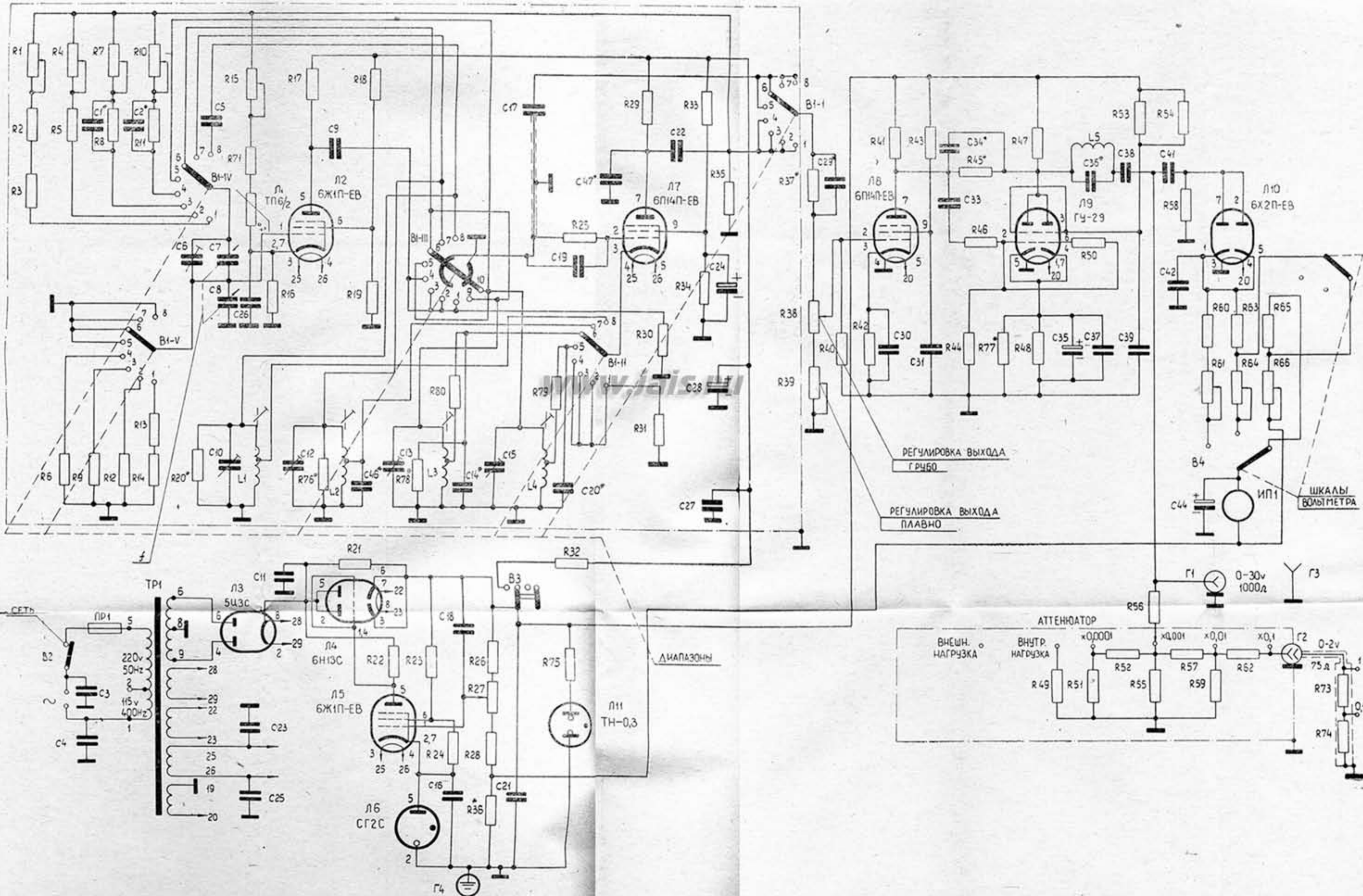
Черт. 6. Схема принципиальная электрическая ГЗ-7А
