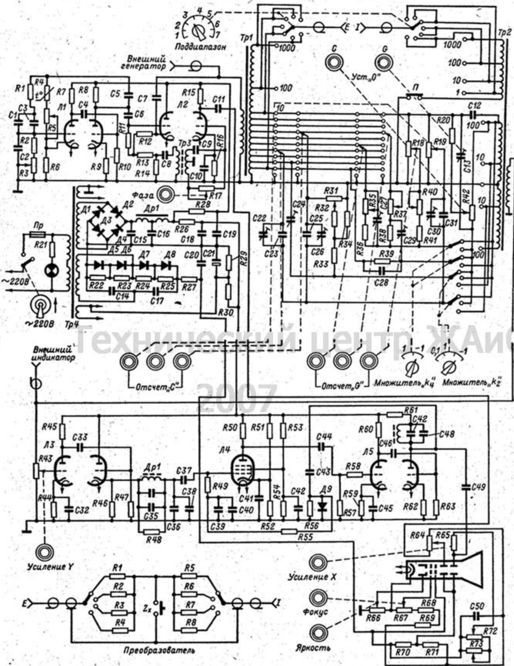
Электрическая принципиальная схема измерителя емкости Е8-2.
