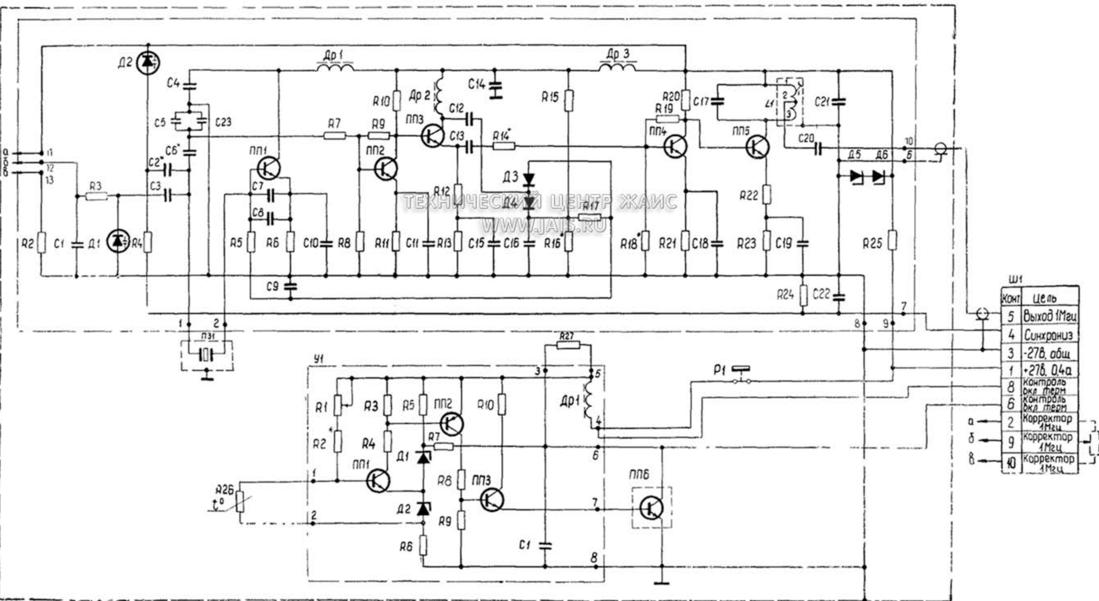
Схема принципиальная электрическая
