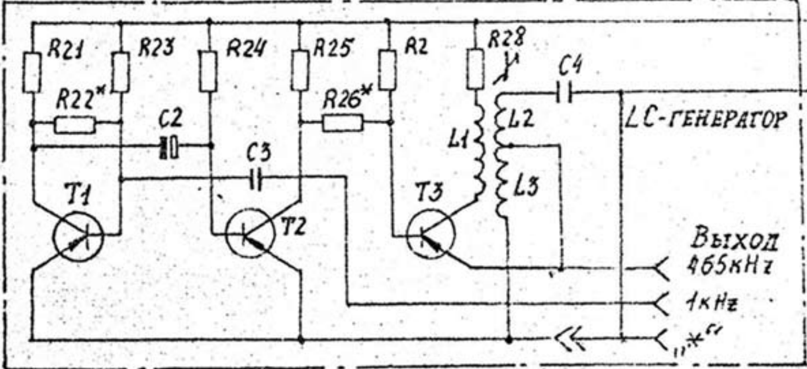
Схема электрическая принципиальная с 04.1973 г.
