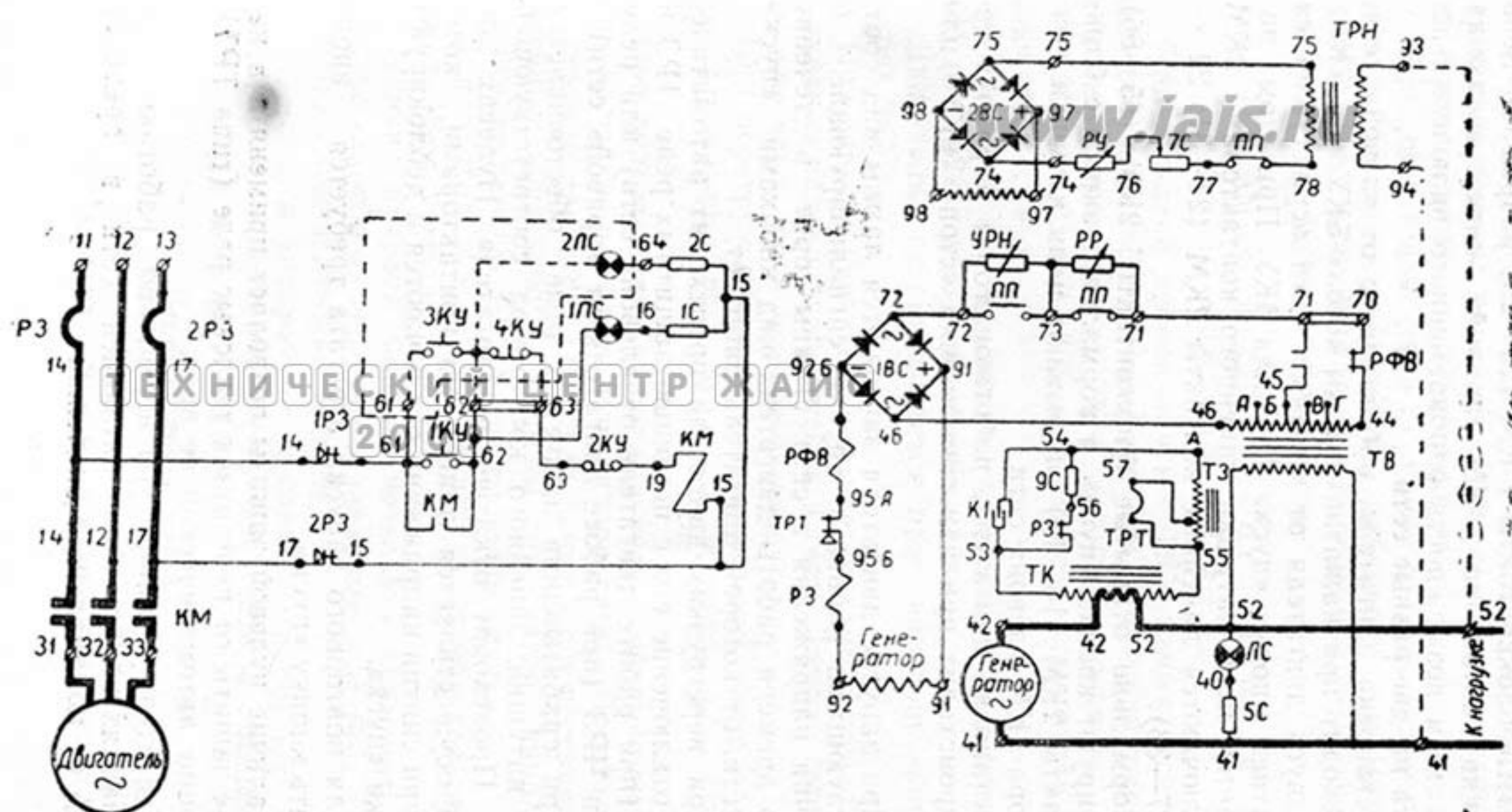
Принципиальная схема агрегата типа АЛА-3,5-М-0
