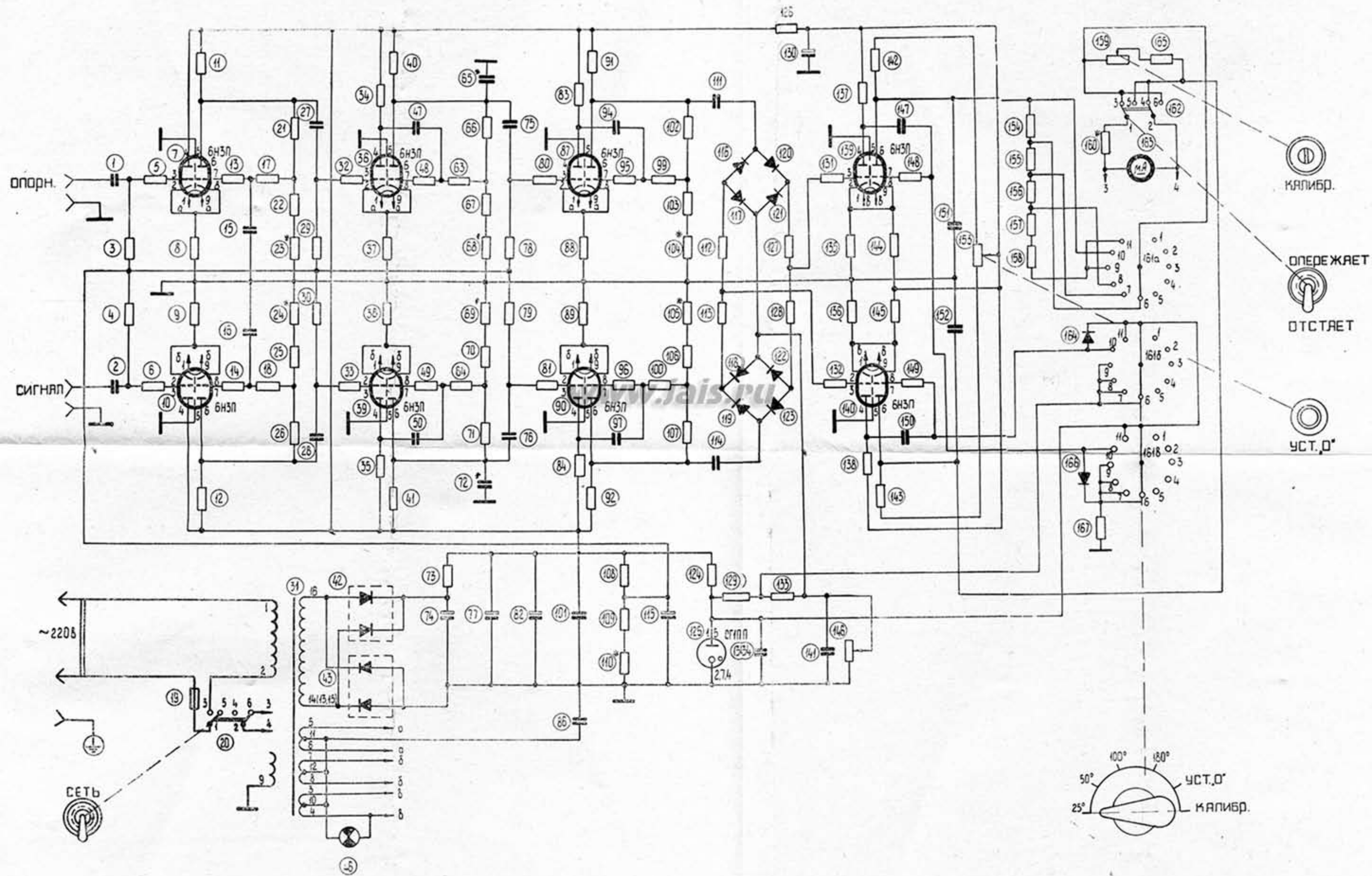
Схема принципиальная электрическая прибора Ф2-1.
