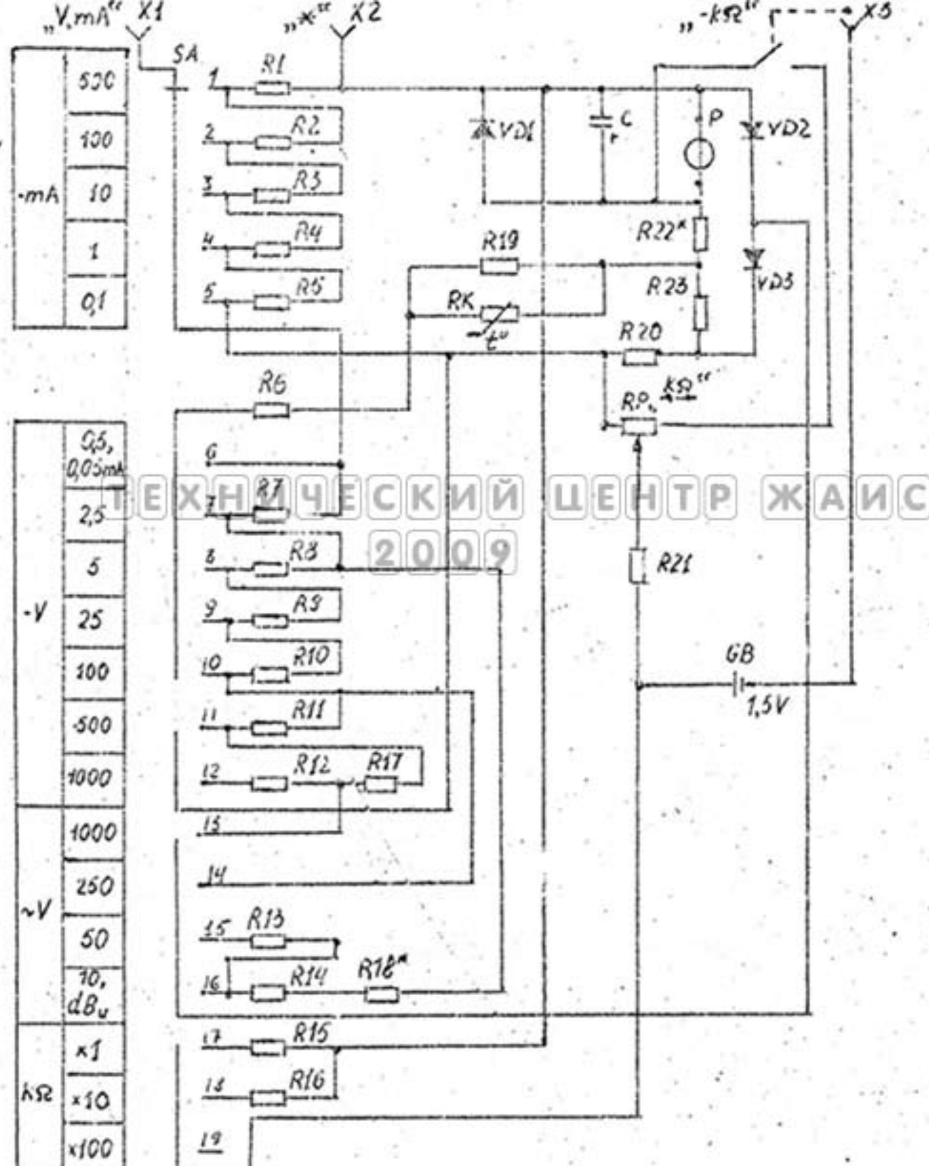
Схема электрическая принципиальная с 01.1985 г.
