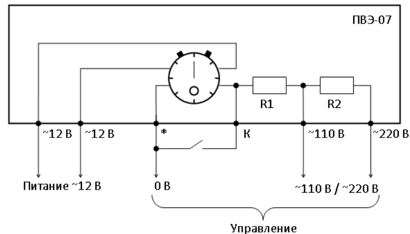
Рис. 4.1. Схема управления секундомером электронным ПВЭ-07
