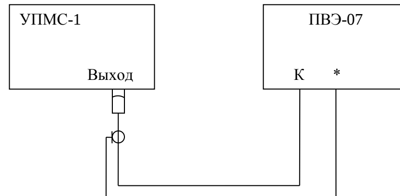
Рис.10.1. Схема подключения приборов при определении погрешности секундомера
